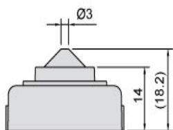
PINHOLE LENS(P4)
